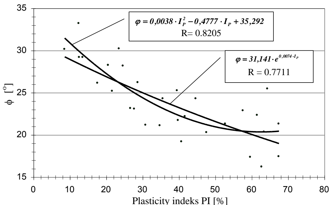
Slika 5.9. Korelacija kuta trenja s indeksom plastičnosti prirodnih materijal, (iz literature)
