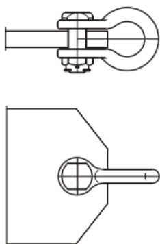
Slika 3.25. Zavješanje za zatezne izolatorske lance sa škopcem
