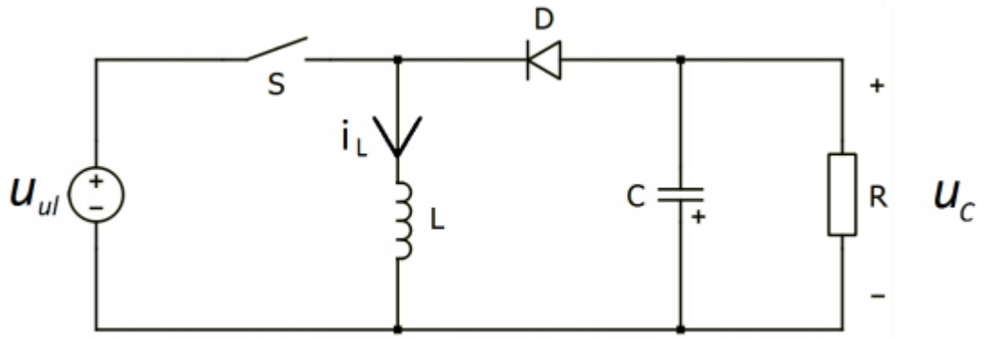
Slika 5.8. Električna shema silazno-uzlaznog DC pretvarača
