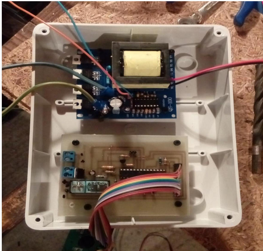
Slika 6.12. Unutrašnjost uređaja
