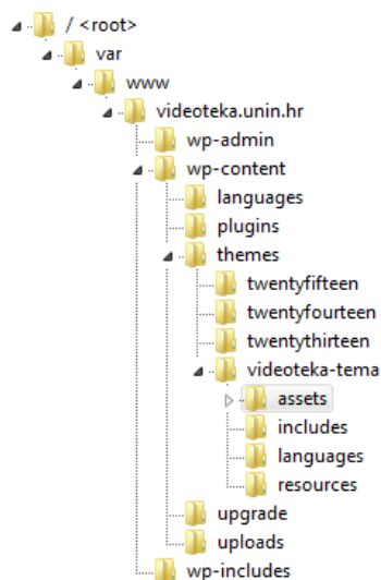
Slika 6-11 Hijerarhijski raspored datoteka
