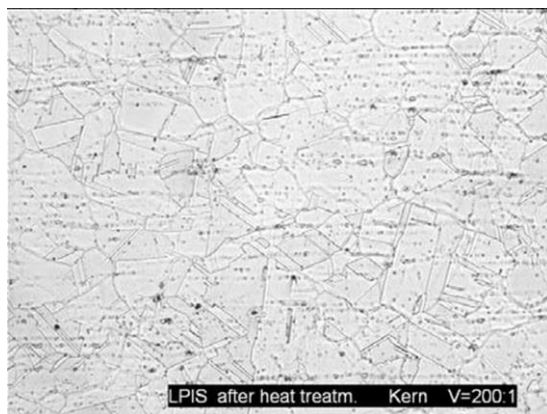
Slika 7.11 Presjek mikrostrukture materijala LPIS na srednjoj zoni nakon toplinske obrade 1170°C / 10 min / voda V = 100:1 60ml HCL / 10 ml HNO 3
