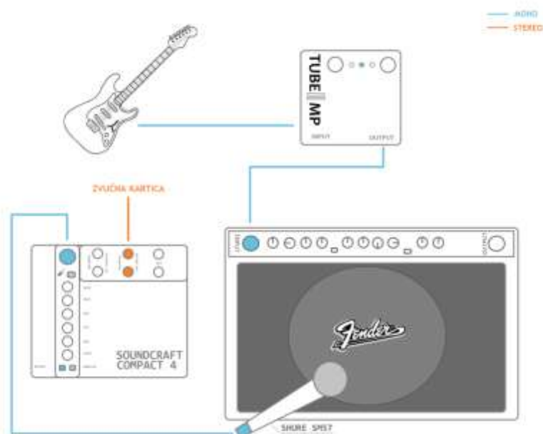
Slika 13. shematski prikaz gitare u spoju s pretpojačalom, pojačalom i miješalom.
