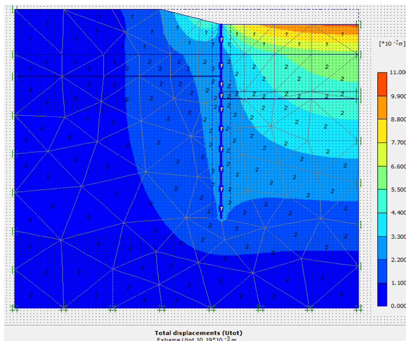
Slika 16. Pomaci tla nakon manjeg iskopa i zabijanja žmurja
