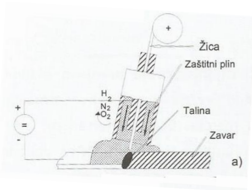
Slika 3.1. MAG zavarivanje[13]
