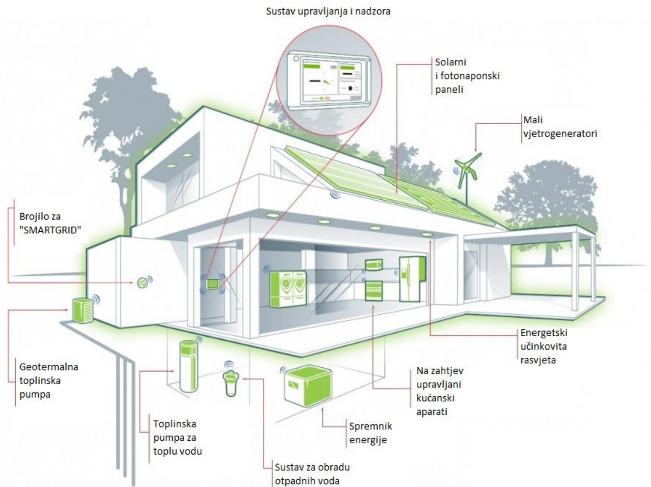
Slika 3.2. Energetske komponente „Zero energy“ kuće
