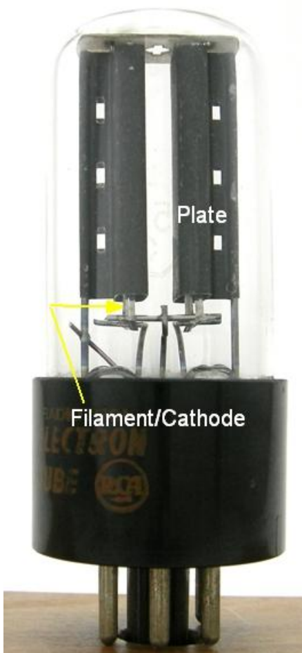
Slika 2.7. 5Y3GT ispravljačka cijev [2]
