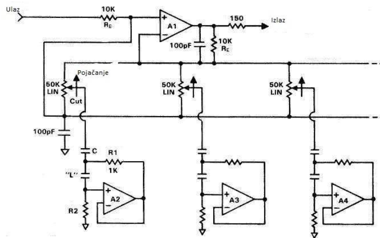
Slika 3.18. Shema spoja [10]
