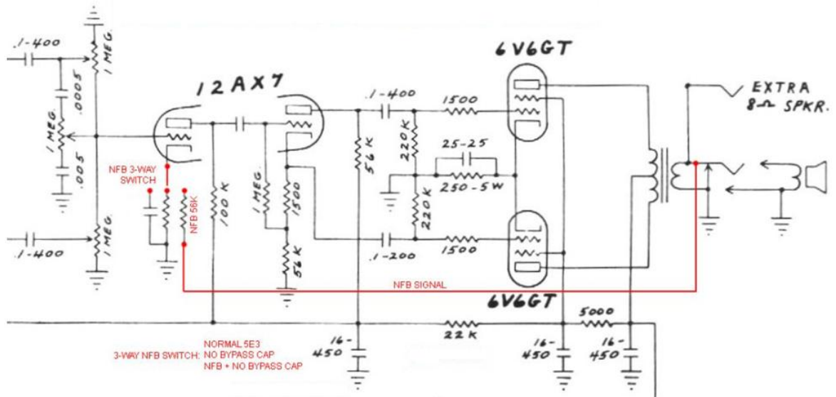
Slika 3.11. Shema spoja; Otpornik od 56\text{k}\Omega je za zvučnik od 8\Omega . Zamjenom s manjom vrijednosti dobiva se veća količina povratne veze. [7]
