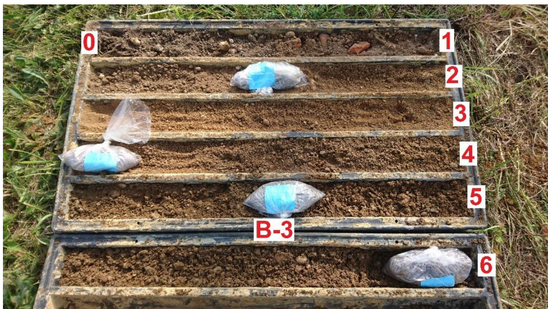
Slika 4.9. Jezgra bušotine B3
