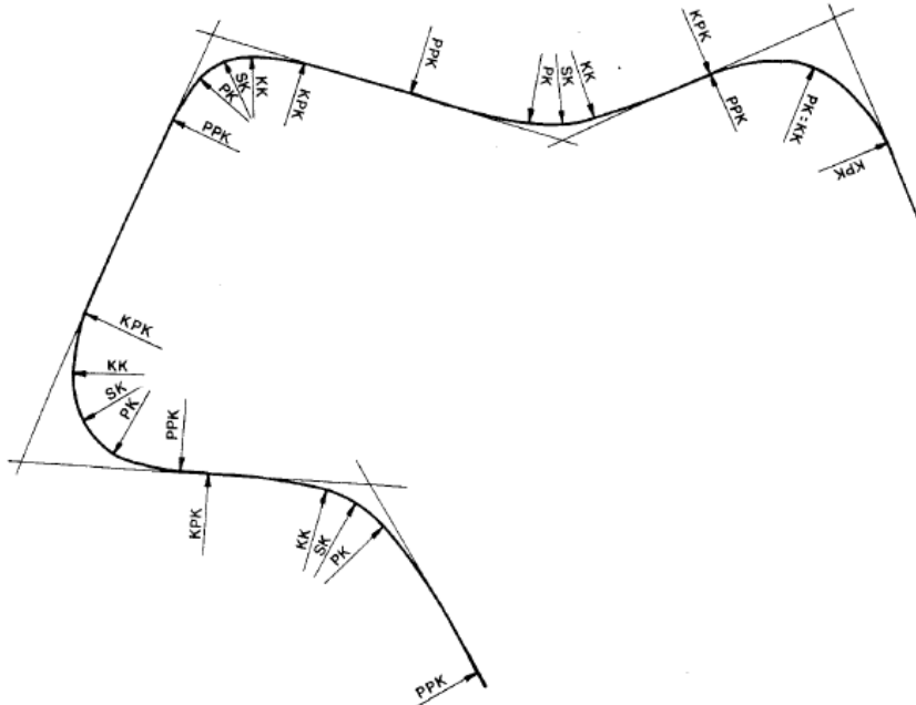
Slika 5.1: Tlocrtni elementi trase (Rezo, 2016.)
