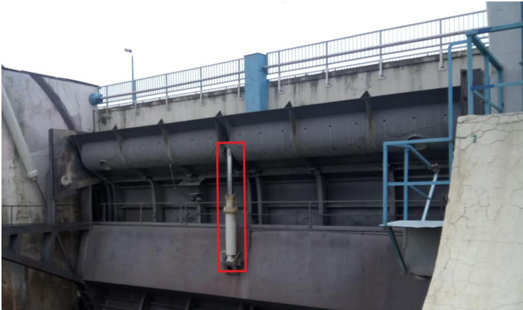
Slika 2.8. Preljevno polje, Servomotor zaklopke
