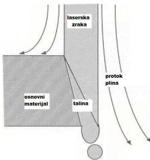
Slika 5.2 Lasersko rezanje taljenjem [14]
