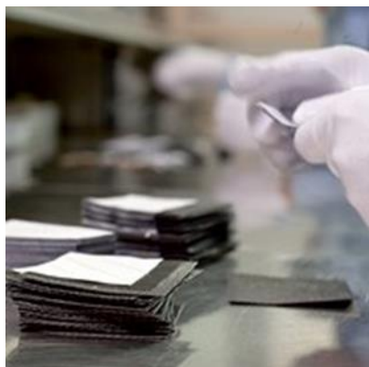
Slika 3.13 Priprema slojeva karbona [11]
