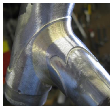
Slika 3.3 Spoj cijevi spojom čahurom i tvrdim lemljenjem [7]
