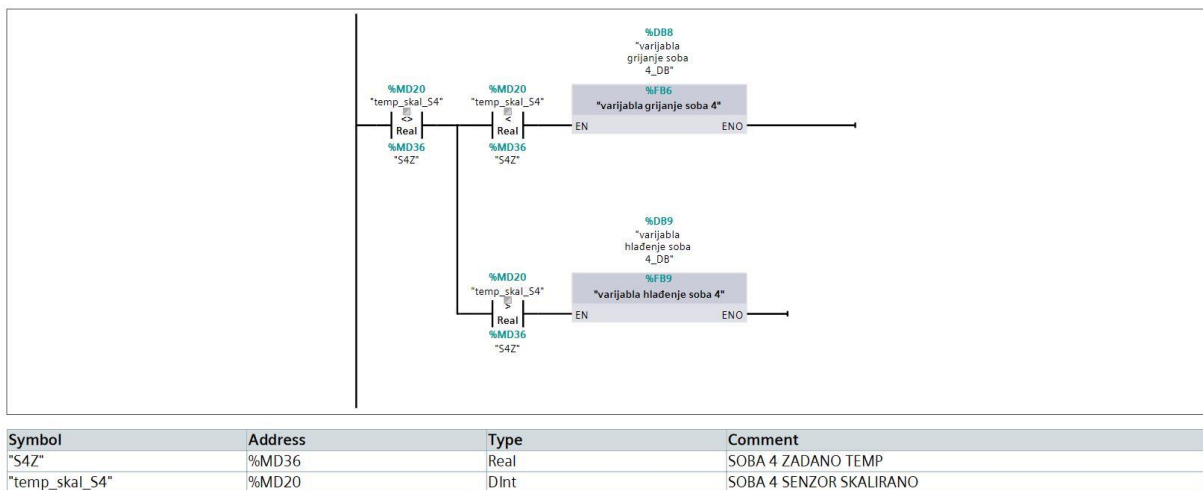
Slika 6.5.3.15. Potprogram Odluka – Network 8
