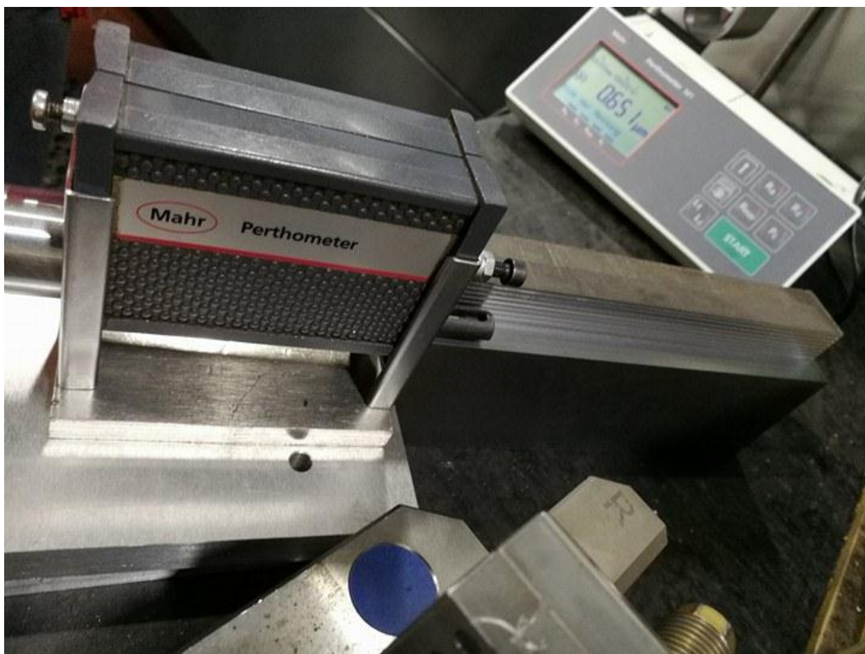
Slika.4.9 Uređaj za mjerenje hrapavosti korišten u testiranju.
