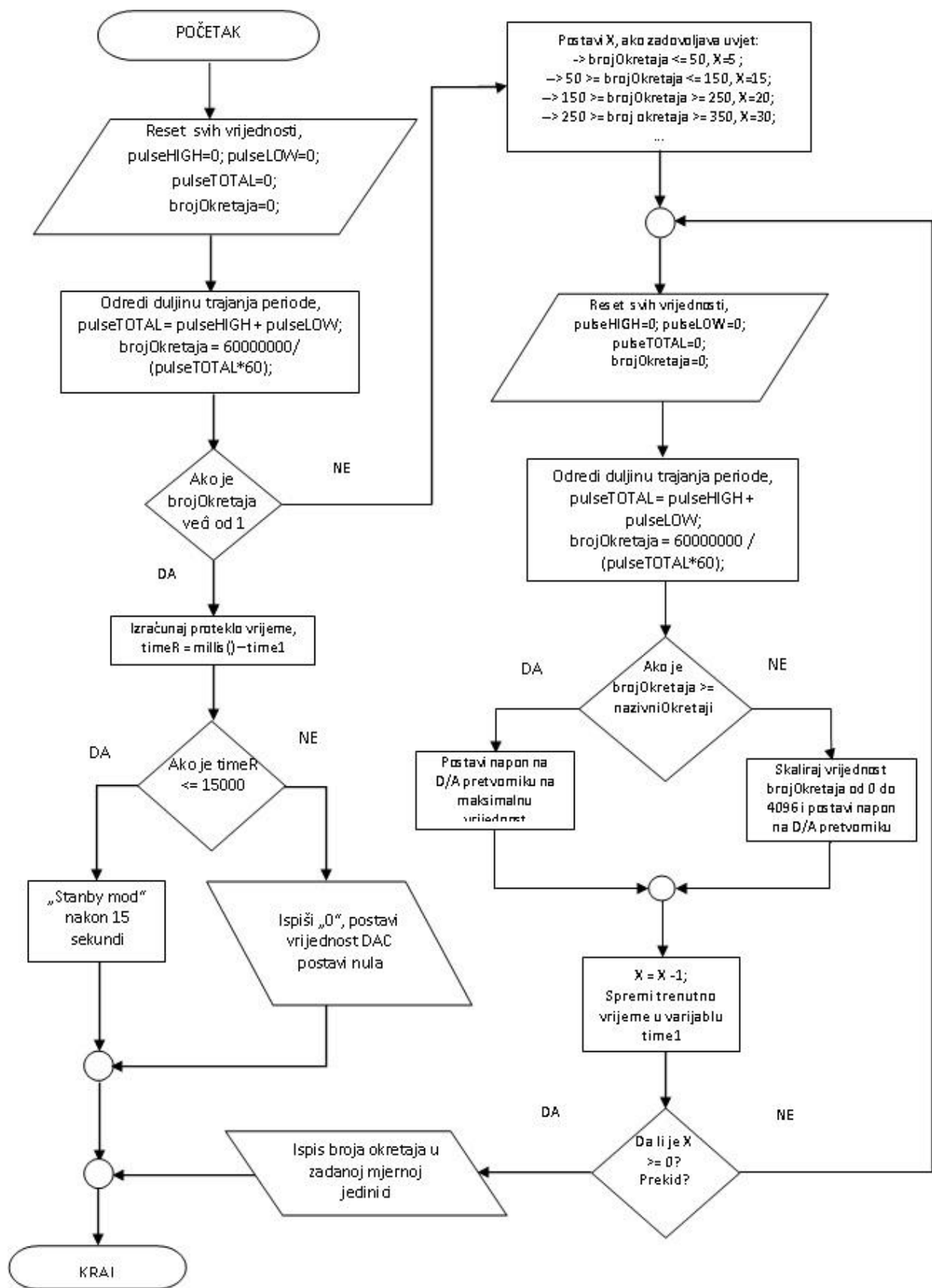
Slika 22. Dijagram toka funkcije mjerenja i prikaza broja okretaja
