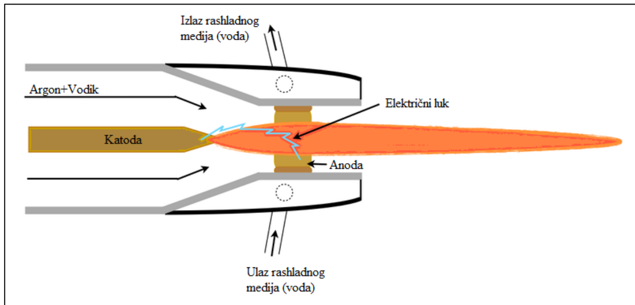
Slika 5.3. Plazma plamenik.[12]
