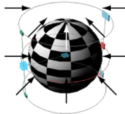
Slika 3.8. Cilidrično mapiranje [30]
