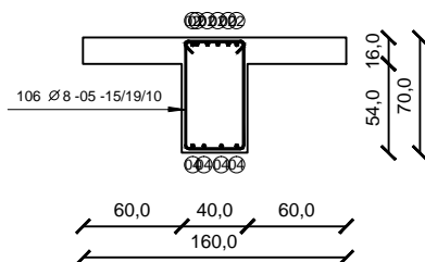
Presjek: B-B
