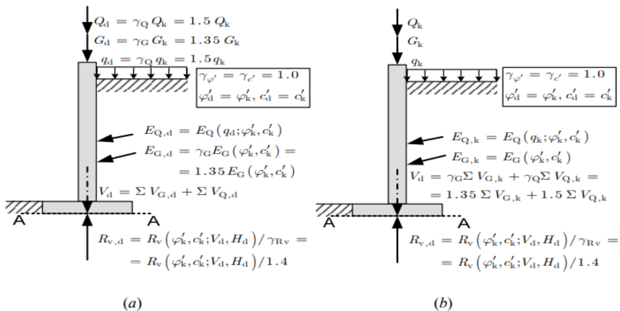
Slika 23: Projektni pristup 2
