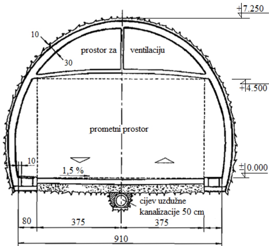
Slika 2.9. Presjek tunela Mala Kapela
