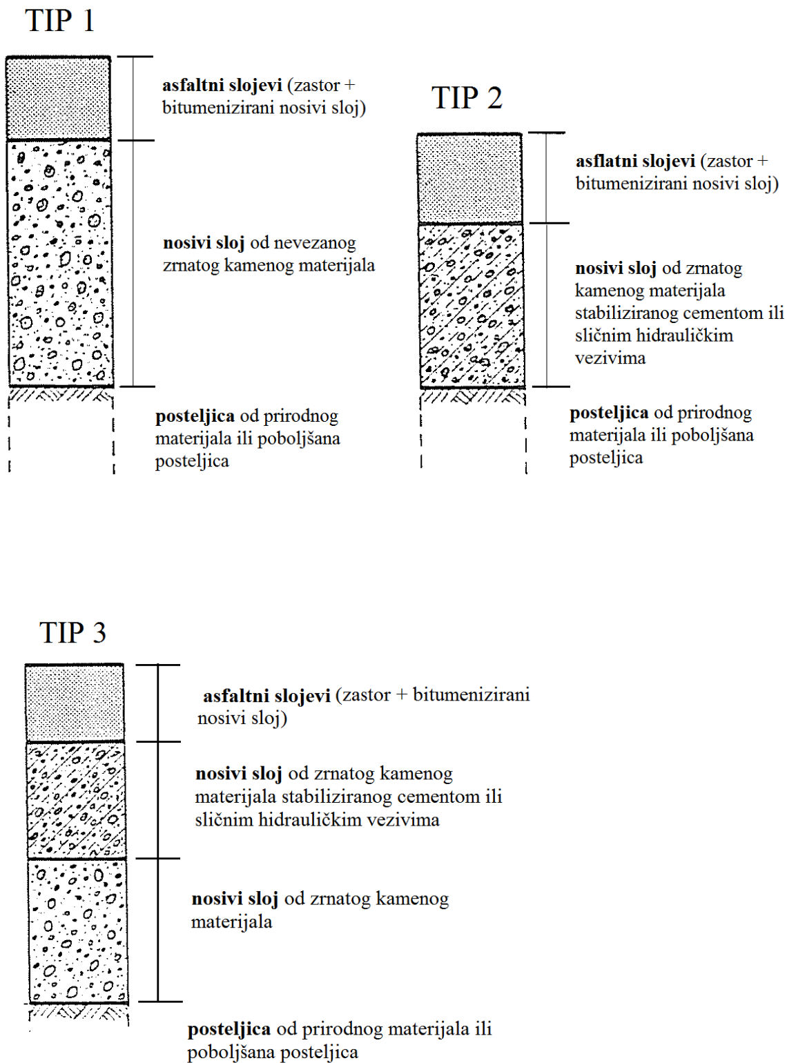
Slika 3.6., 3.7., 3.8. Tipovi rješenja kolničkih konstrukcija po HRN-metodi
