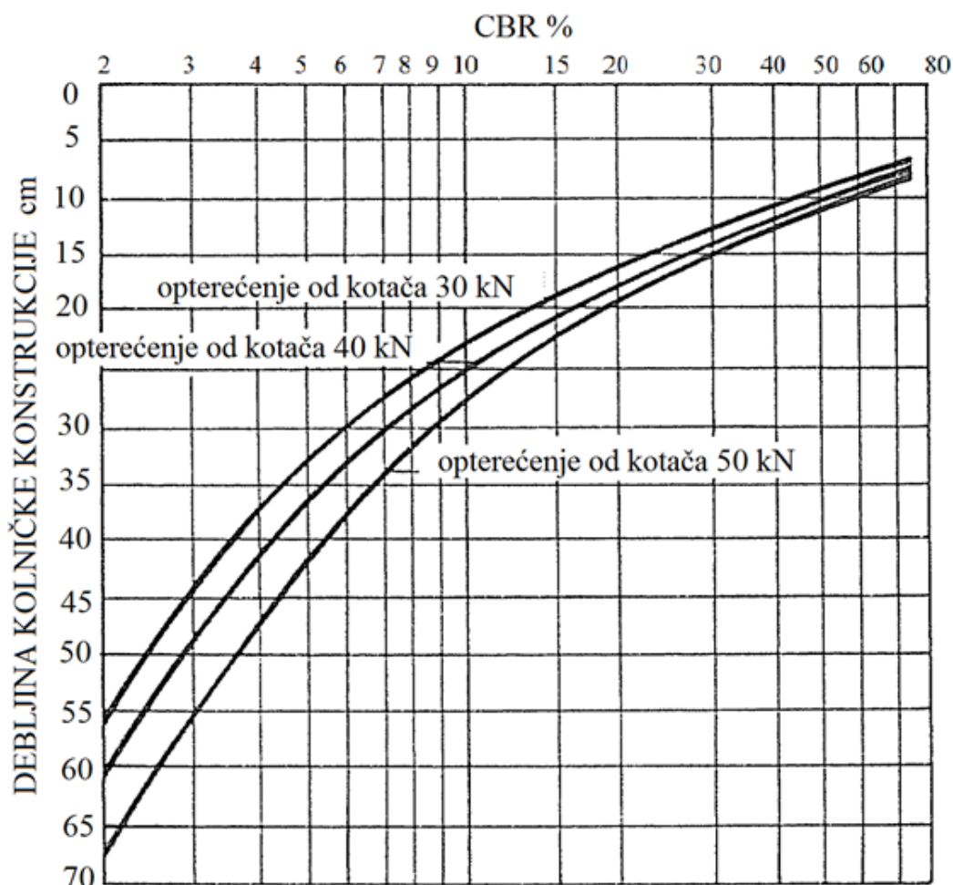
Slika 3.1. Dijagram za dimenzioniranje kolničkih konstrukcija po CBR metodi
