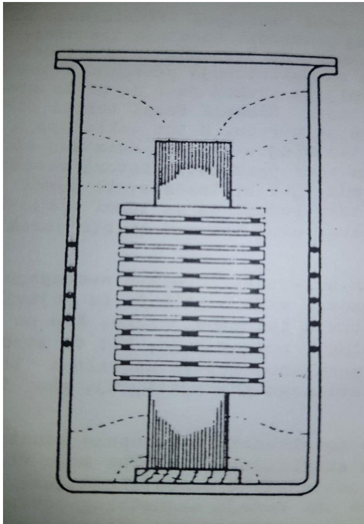
Slika 2.5.1. Uljni transformator[2]
