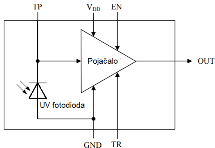
Slika 2.11. UV senzor[13]
