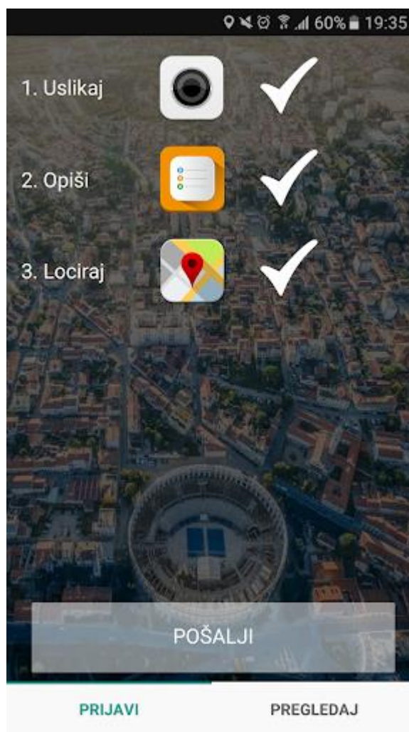
Slika 16. Aplikacija SmartPula
