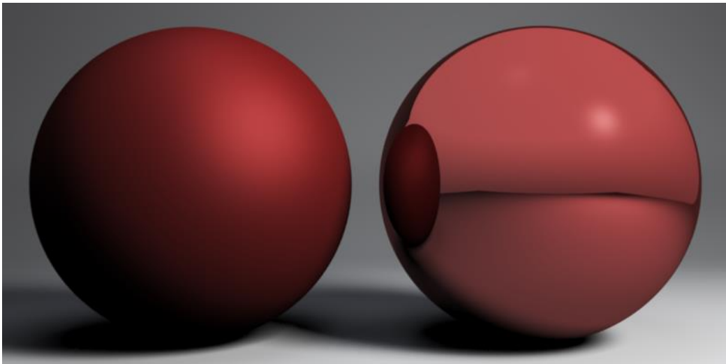
Slika 3.26 Refleksije modela [8]
