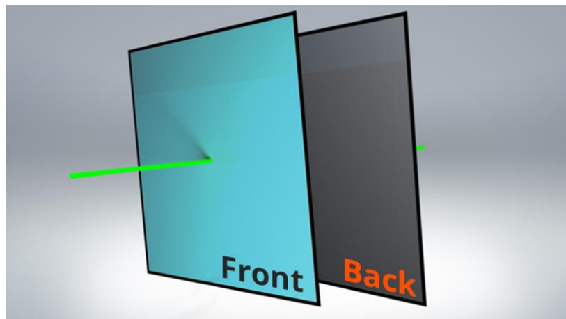
Slika 3.27 Normale [7]
