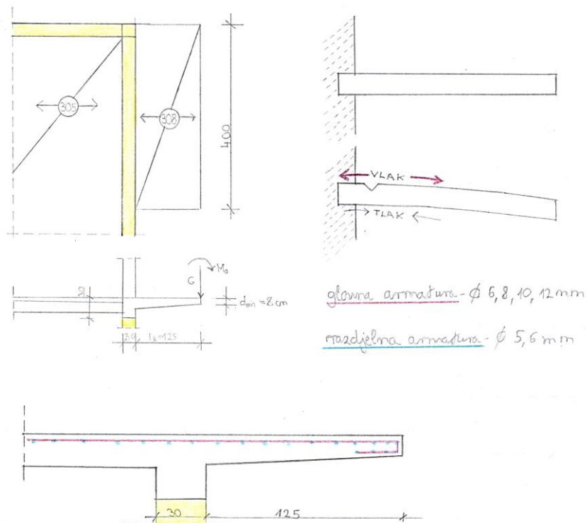
Slika 2.3 Konzolna ploča
