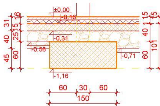
TEMELJ T3 i T4
