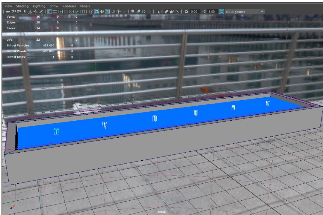
Slika 10.41 Kopiranje
