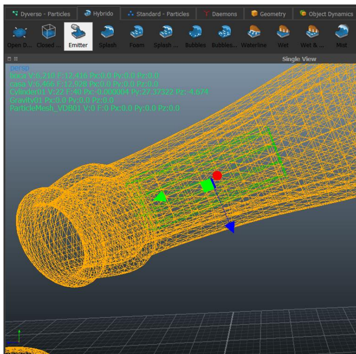
Slika 10.15 Emitter
