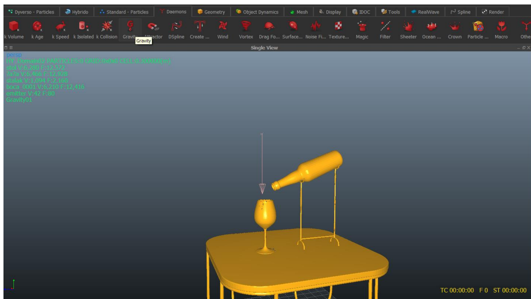
Slika 10.17 Postavljanje gravitacije
