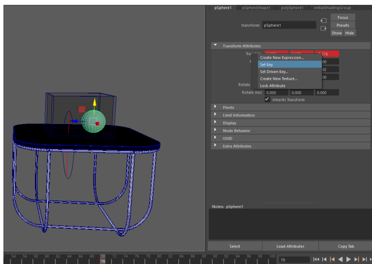
Slika 10.28 Animiranje kugle
