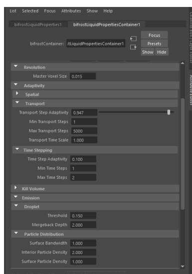
Slika 10.30 Postavke emisije
