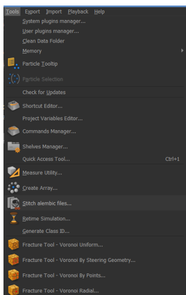
Slika 10.22 Spajanje datoteka
