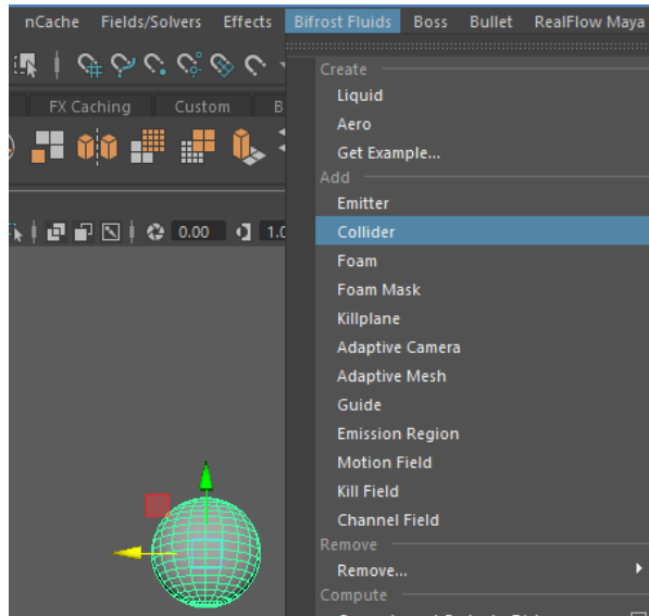
Slika 10.27 Collider
