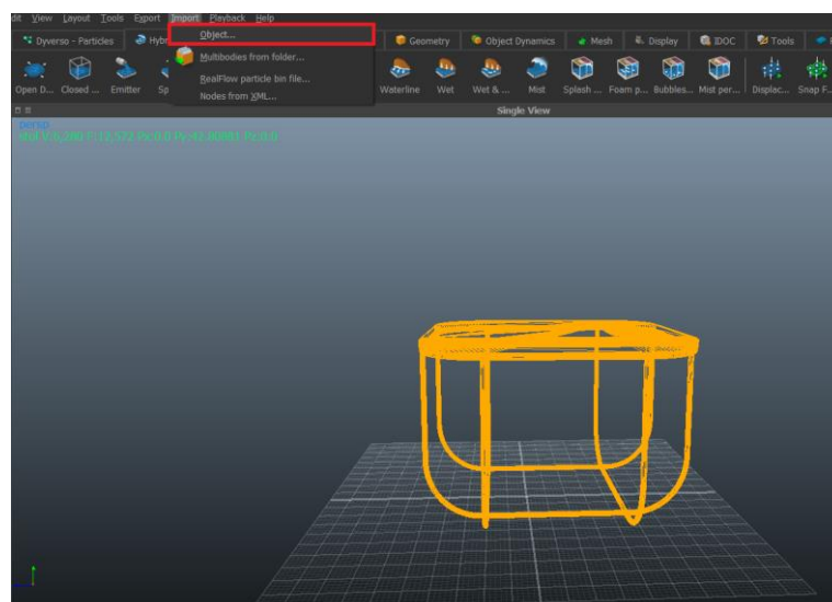
Slika 10.14 Import
