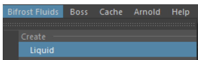
Slika 10.4 Stvaranje tekućine
