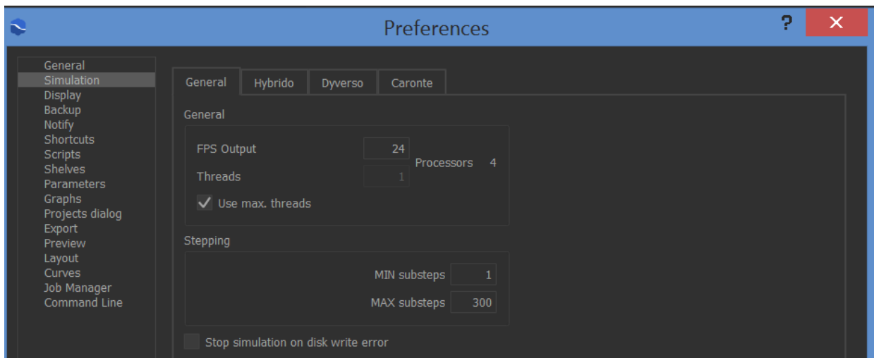
Slika 10.13 Postavke simulacije
