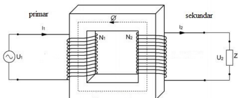
Slika 3.7 Shema transformatora
