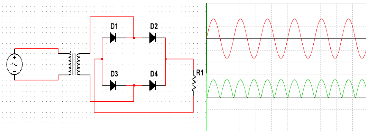
Slika 4.5 Shema spoja punovalnog ispravljača pomoću Grectzovog spoja i izgled ispravljenog napona
