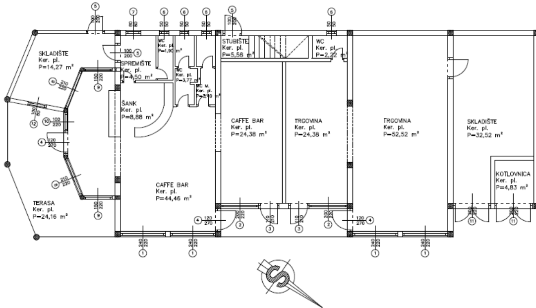
Slika 3 Tlocrt prizemlja
