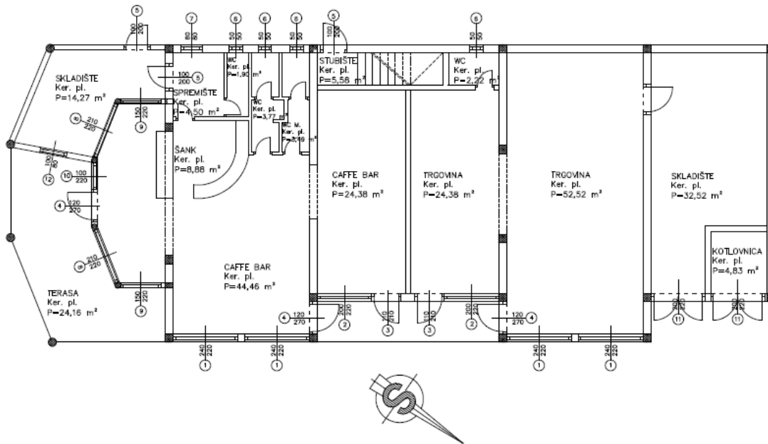
Slika 3 Tlocrt prizemlja
