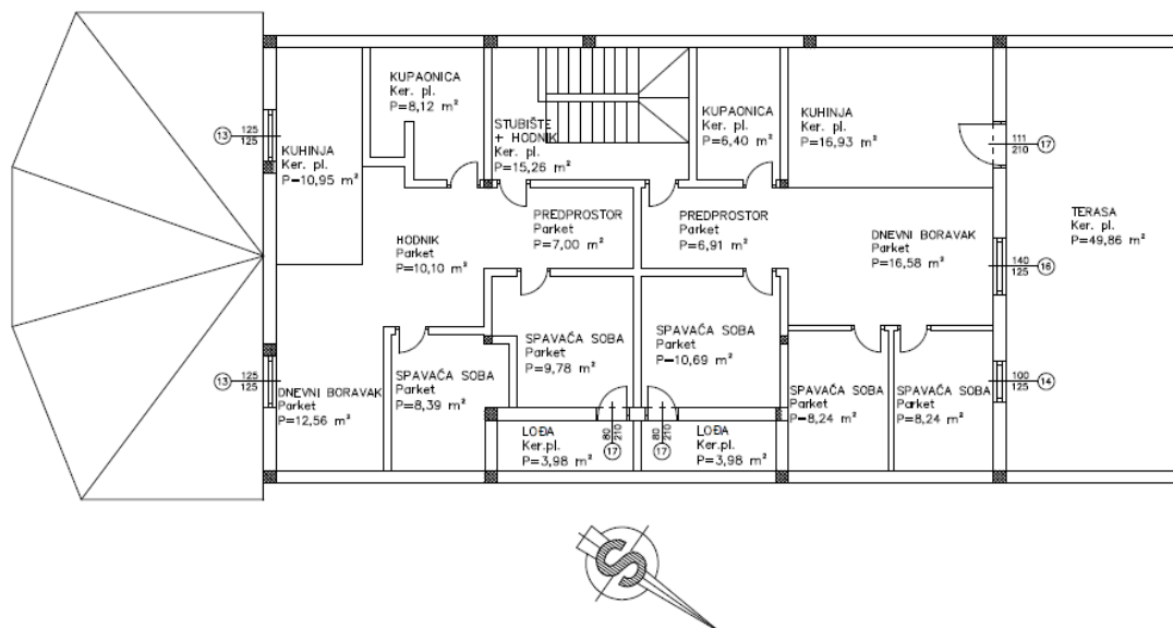
Slika 4 Tlocrt kata
