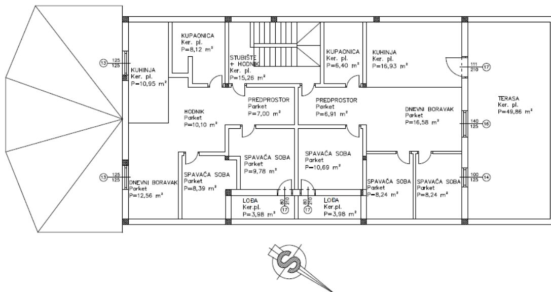
Slika 4 Tlocrt kata
