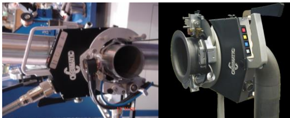
Slika 7.4.3. Otvorena glava sa AVC kontrolom (lijevo) i bez AVC kontrole (desno).[36]
