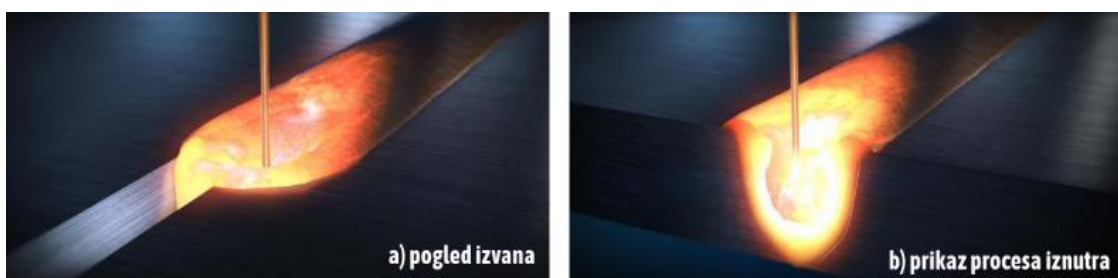
Slika 5.7.1. Prikaz metode zakopanog luka.[23]
