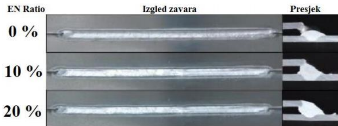
Slika 5.5.1. Utjecaj negativnog polariteta pri spajanju aluminijske legure (AC MIG).[7]
