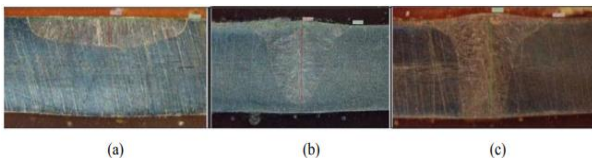
Slika 7.2.2. Utjecaj aktivirajućeg praška na protaljšivanje kod TIG zavarivanja.[8]
