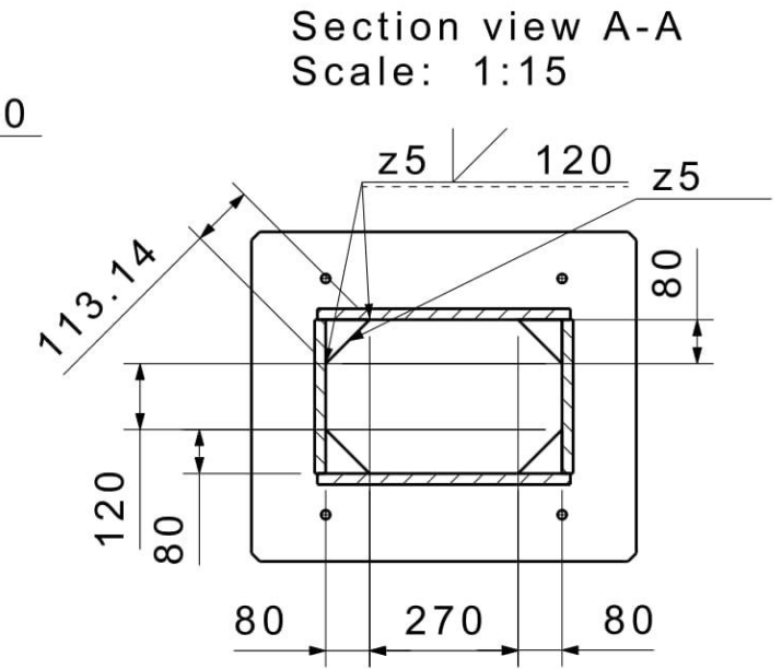
Section view A-A Scale: 1:15
