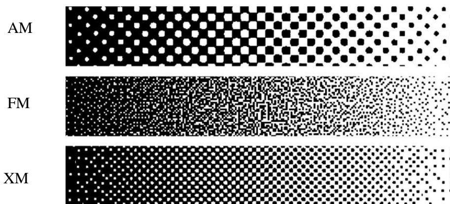
Slika 12. Podjela rastera
