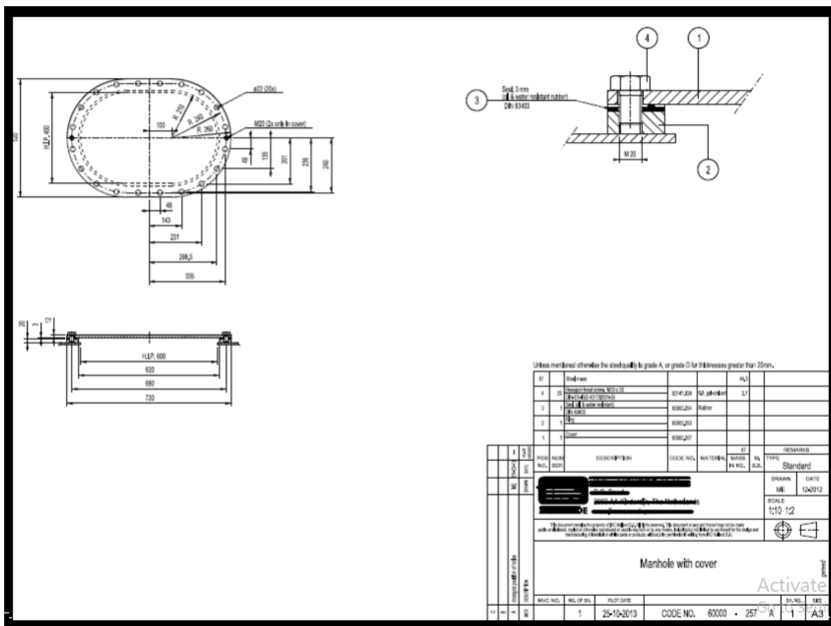
Slika 17. Primjer nacrt za proizvodnju
