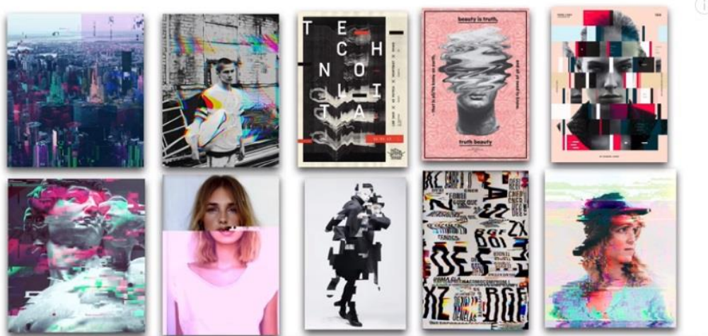
Slika 3.1 Glitch efekt
