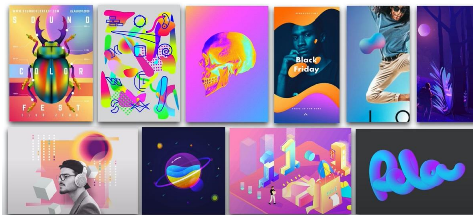
Slika 3.5 Električni gradijent
