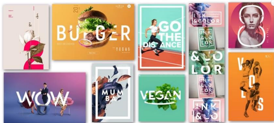
Slika 3.3 Integracija grafike
