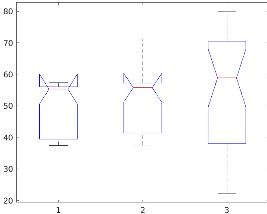
Slika 6.94 - Prikaz ANOVA dijagrama za BRISQUE metodu.
