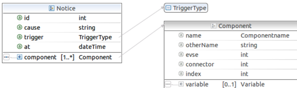
Slika 6.2. "Notice" struktura [1]
