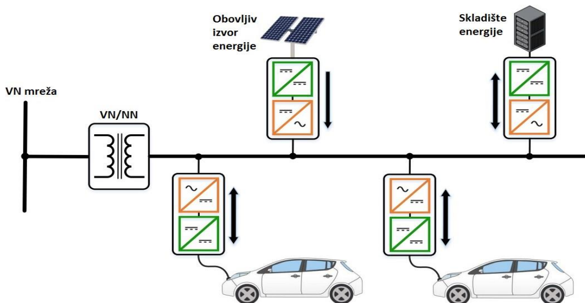
Slika 3.3. AC sabirnica za brzo punjenje [7].
