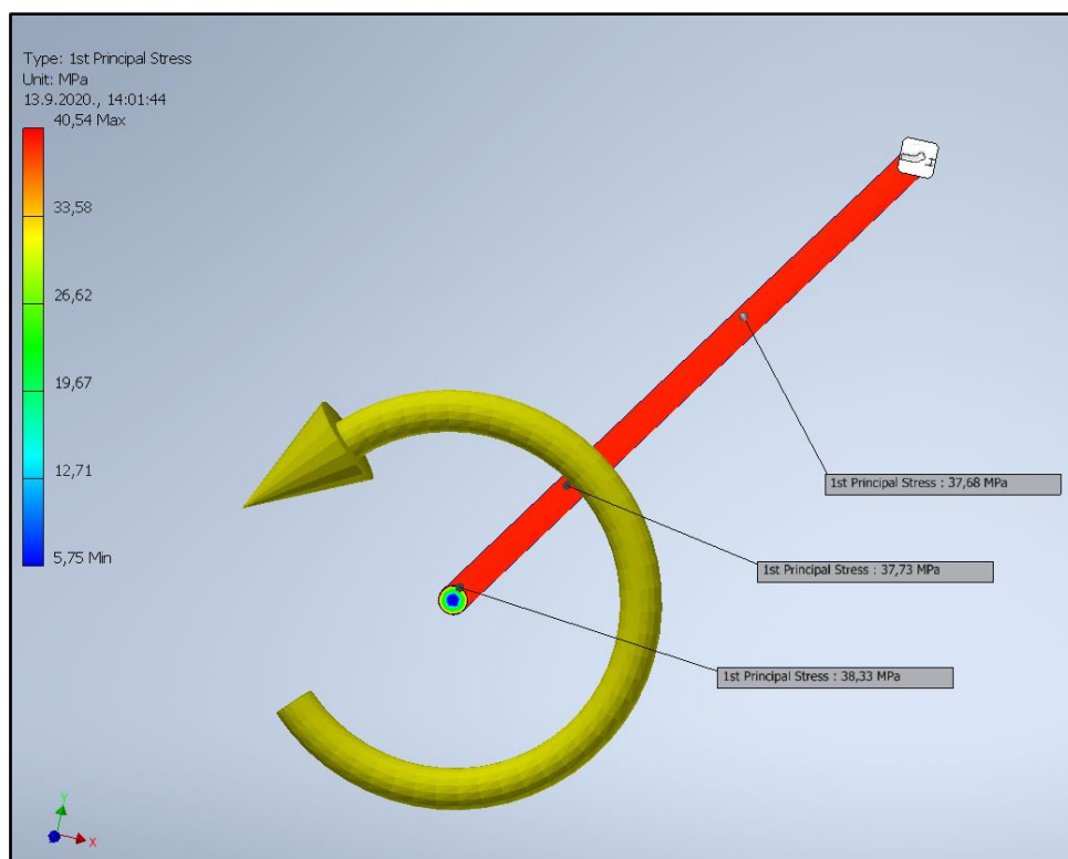
Slika 5.7 Maksimalna tangencijalna naprezanja za zadatak 5.1.
