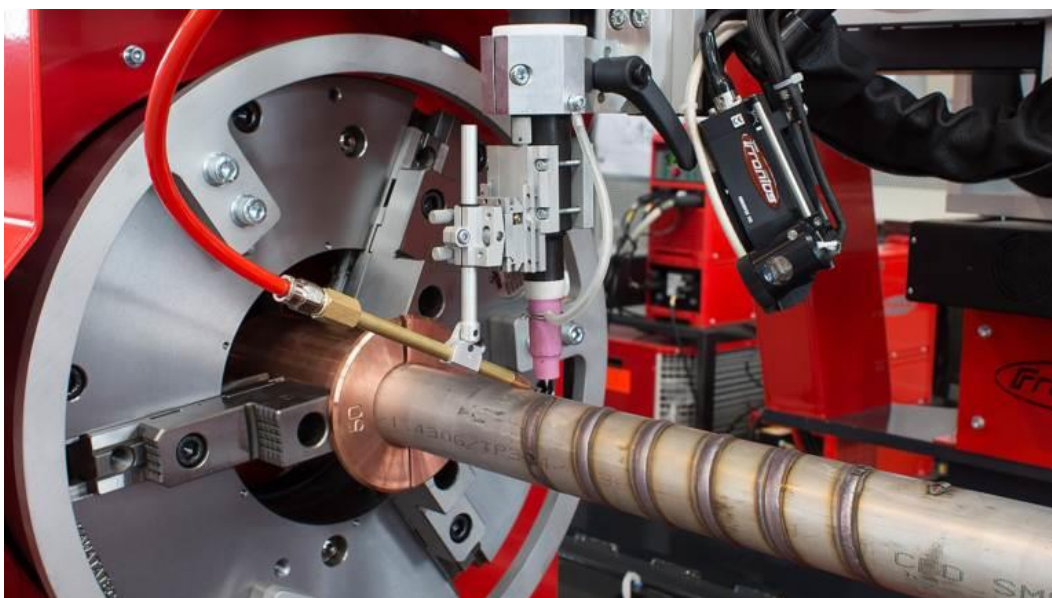
Slika 2.30 Spiralni zavar [34]
