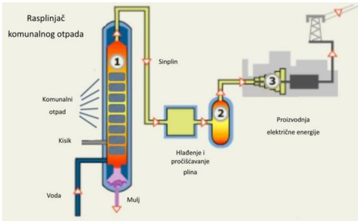
Slika 8. Shema rasplinjavanja [10]
