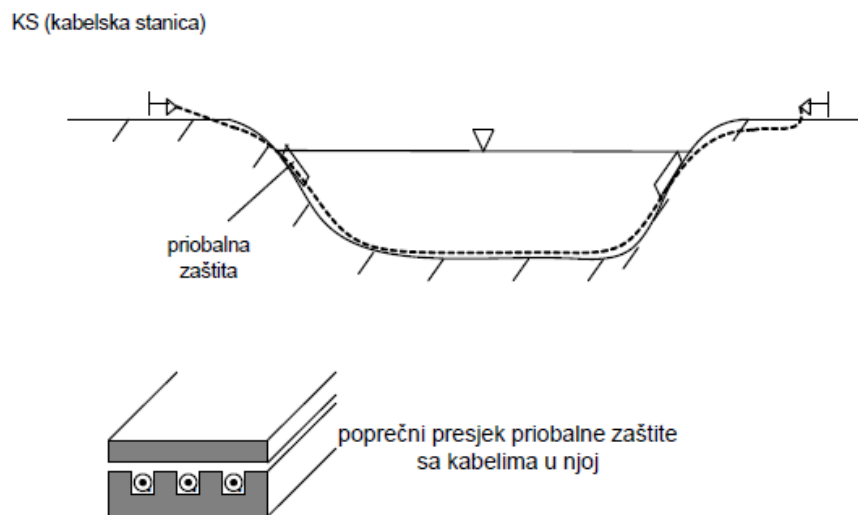
Slika 3.15 Polaganje kabla
