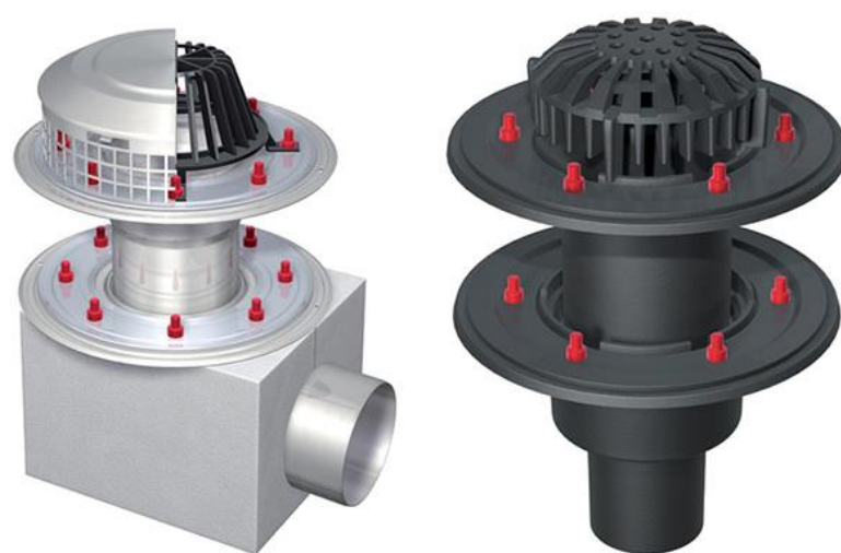
Slika 27. Slivnici za odvodnju vode na ravnom krovu
