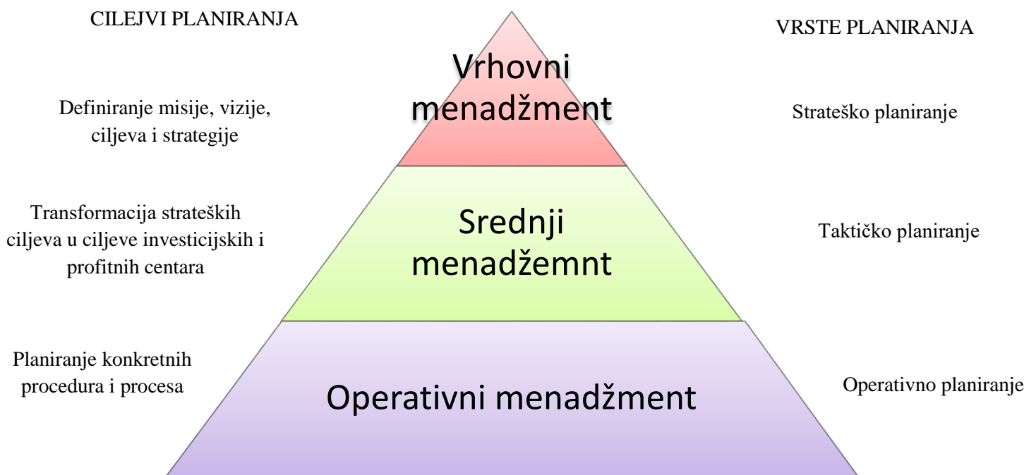
Slika 2.2. Vrste planova prema hijerarhiji, Belak (2014.)
