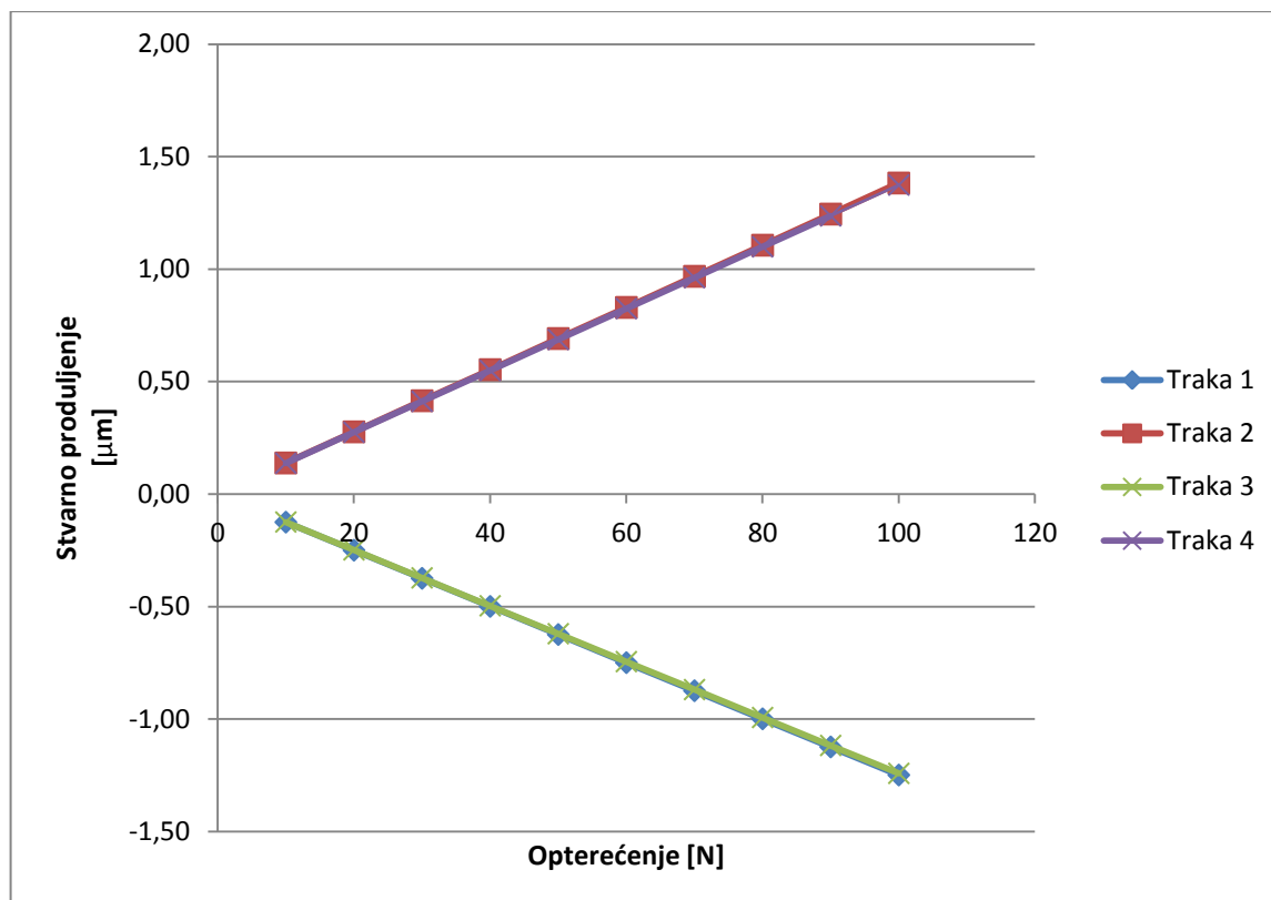
Slika 5.6 Stvarno produljenje
