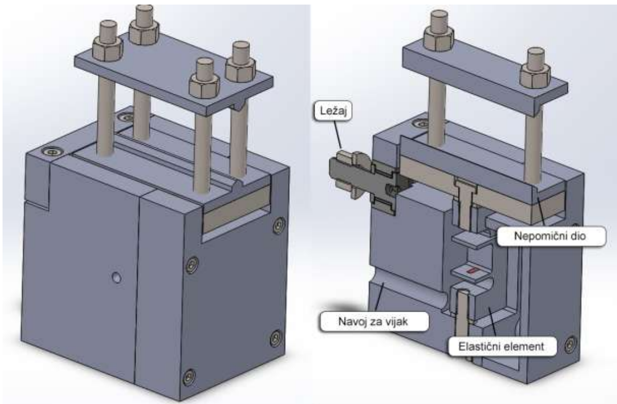
Slika 4.12 Druga varijanta oslonca (nepomični oslonac)
