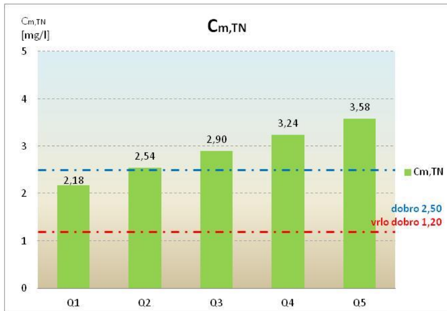
Slika 5.12. Grafički prikaz koncentracija TN nakon miješanja preljevni voda i protoka kroz akumulaciju u ovisnosti dinamici rada crpki crpne stanice za preljevne količine
