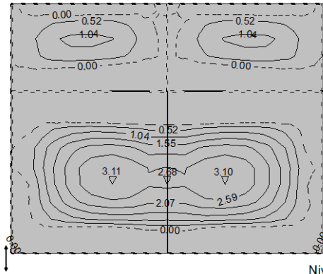
Nivo: [4.40 m] Aa - d.zona - Pramac 2 - max Aa2,d= 3.11 cm 2 /m
