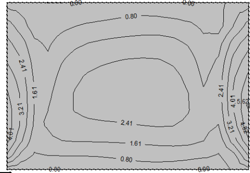
Okvir: V_3 Aa - d.zona - Pramac 1 - max Aa1,d= 5.62 cm²/m
