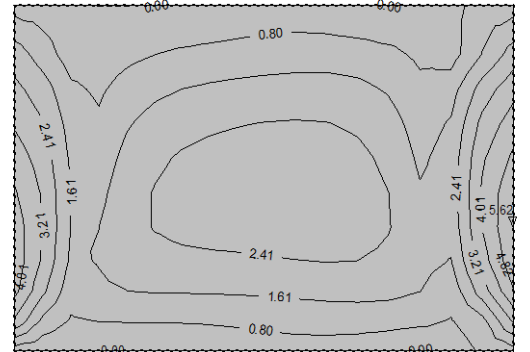
Okvir: V_3 Aa - d.zona - Pramac 1 - max Aa1,d= 5.62 cm 2 /m
