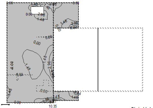
Okvir: V_1 Aa - d.zona - Pramac 1 - max Aa1,d= 10.35 cm 2 /m
