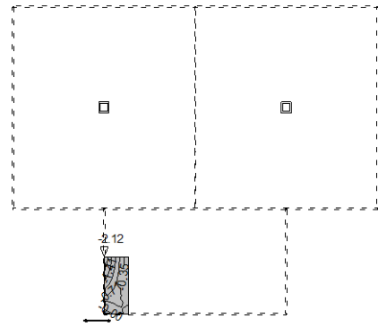
Nivo: [-1.43 m] Aa - g.zona - Pramac 1 - max Aa1,g= -2.12 cm 2 /m
