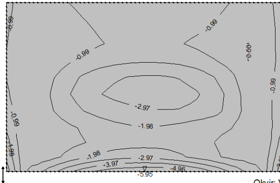
Okvir: V_3 Aa - g.zona - Pramac 2 - max Aa2,g= -5.95 cm 2 /m
