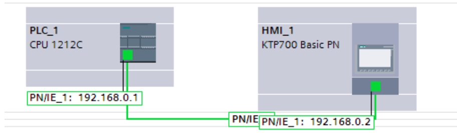
Slika 4.1. Topologija mreže
