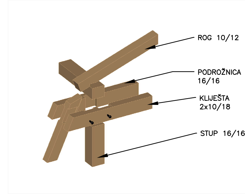
DETALJ 1 M 1:25
