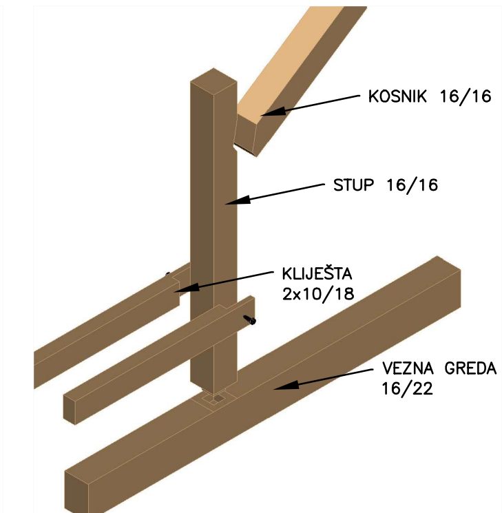
DETALJ 3 M 1:25
