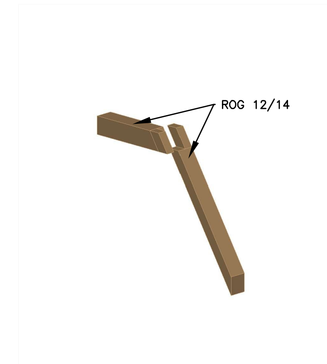
DETALJ 2 M 1:25
