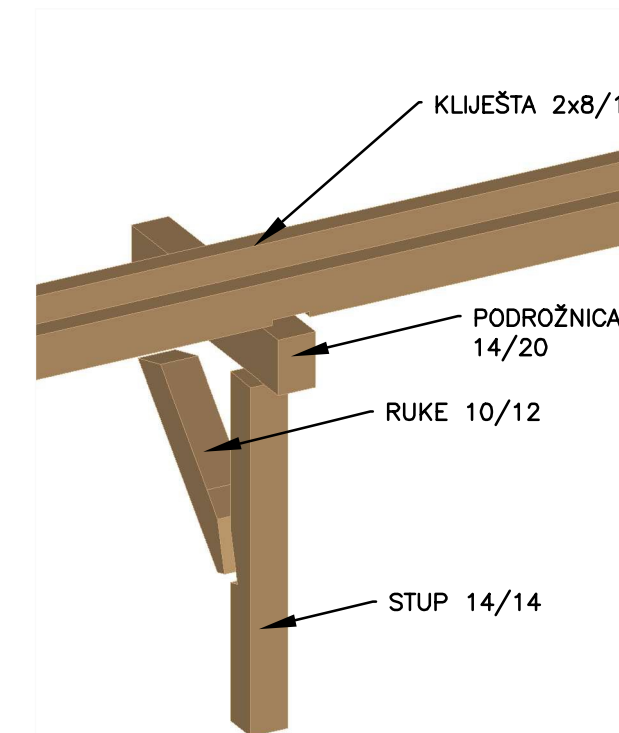
DETALJ 3 M 1:25
