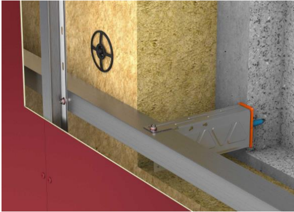
Slika 6.2.4. Montaža potkonstrukcije
